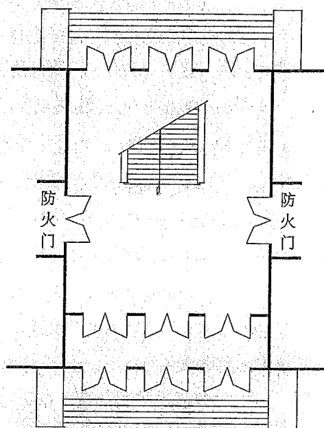
图5 扩大封闭楼梯间示意图
